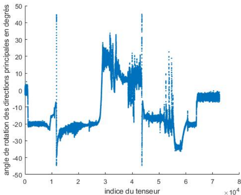
FIGURE 2 – Angle de rotation entre les directions principales dans le plan (0xy) au cours d'un cycle de chargement.
